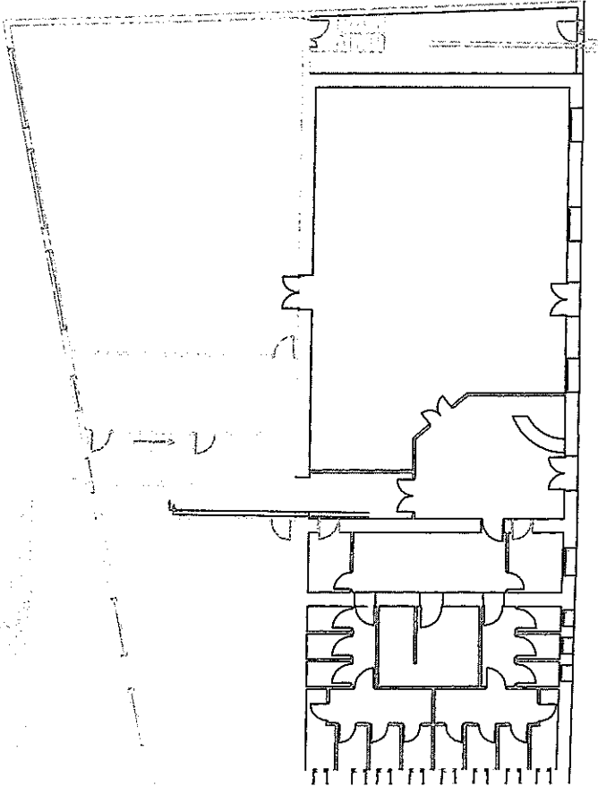
PLAN DE SANITARIO Y FONTANERIA
